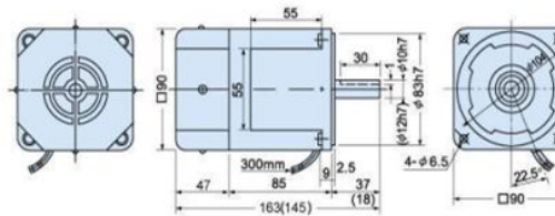
平面鍵: 1×30ℓ
