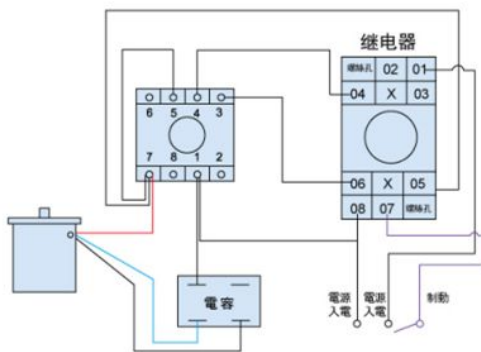
SB31-IN SB32-IN 配線圖
