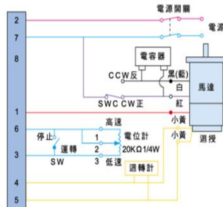
SS31 HR SS32 HR 配線圖
