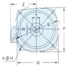
A2-法蘭面
