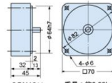
3GN10X 重量: 約0.55kg
