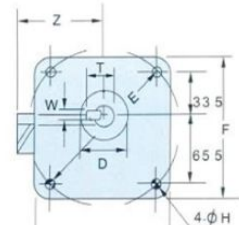
A1-法蘭面
