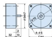
2GN10X 重量: 約0.2kg
