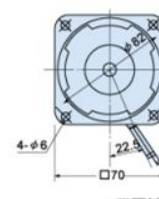
平面鍵: 1×30ℓ
