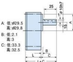
平面鍵: 1×12ℓ
