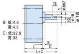
平面鍵: 1×12ℓ
