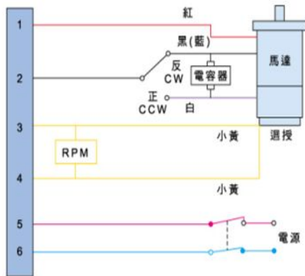
US51 US52 配線圖 UX51 UX52
