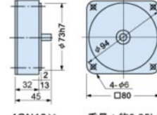
4GN10X 重量: 約0.35kg
